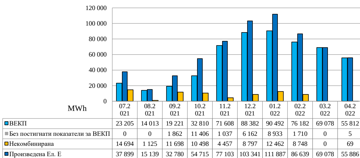
електрическа енергия, произведена от ТЕЦ "София Изток"
