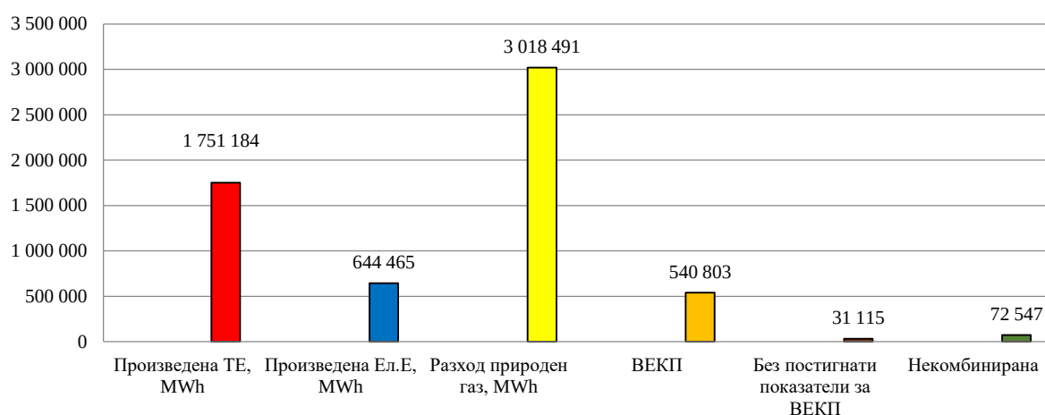
ТИП на ТЕЦ "София Изток" за периода 01.07.2021 г. до 30.04.2022 г.
