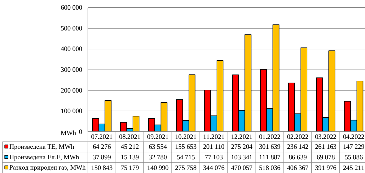
ТИП на ТЕЦ "София Изток" - производствена на електрическа и топлинна енергия и разход на природен газ
